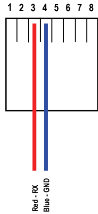
RJ45
